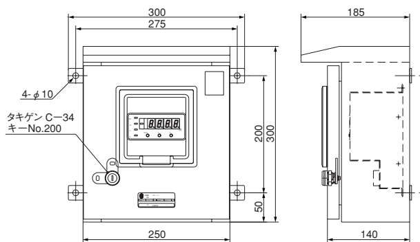
コントロールユニット(屋外設置)
