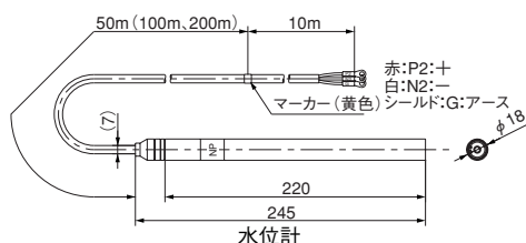
水位計
