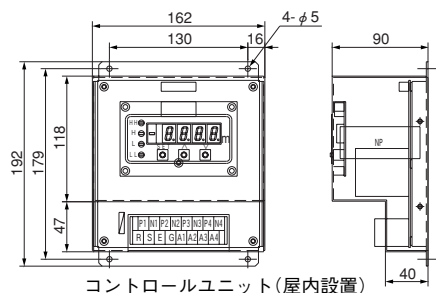
コントロールユニット(屋内設置)
