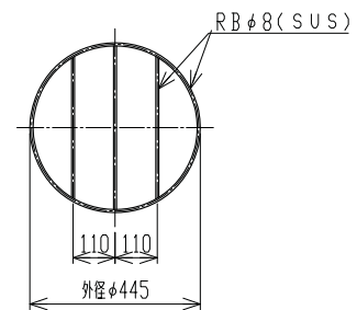
落下防止金具 (オプション)
