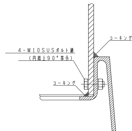
C部断面図
