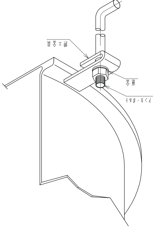
取付要領図
