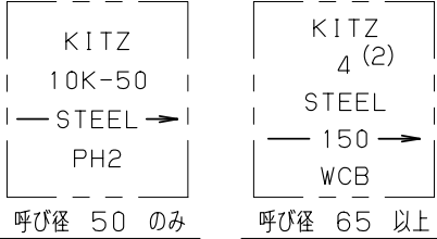
寸法表 単位：mm 呼び径 d H D1 L l フ ラ ン ジ 概算質量 (kg) D ボ ル ト 穴 ボルトの ねじの 呼び g (1) t f C 数 h mm in. D C 数 h g t f 50 2 50.5 332 200 203 20 155 120 4 19 M16 96 16.0 2 21 65 2.1/2 65 379 250 216 21.5 175 140 4 19 M16 116 17.5 2 29 80 3 80 390 250 241 28 185 150 8 19 M16 126 19.1 2 36 100 4 101.5 460 250 292 36 210 175 8 19 M16 151 23.9 2 52 125 5 125 484 300 356 43 250 210 8 23 M20 182 23.9 2 80 150 6 151 513 350 406 49 280 240 8 23 M20 212 25.4 2 91 200 8 203 630 400 495 58 330 290 12 23 M20 262 28.6 2 158
