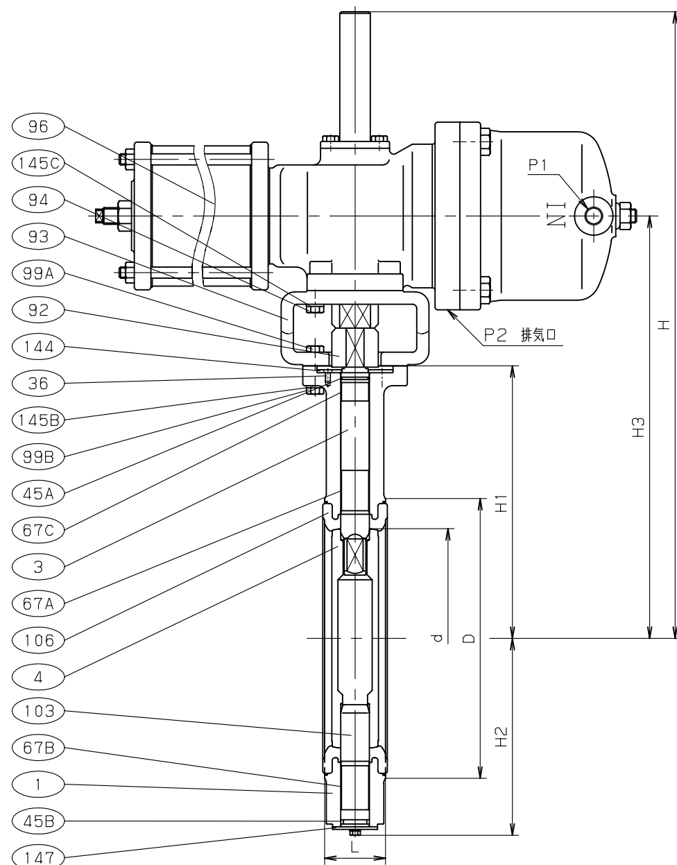
寸法表
