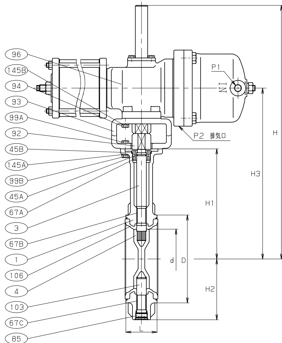
寸法表
