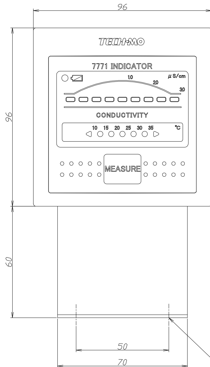
前面図
