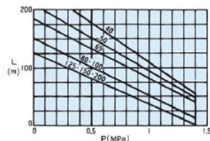
40K形繰出し管
