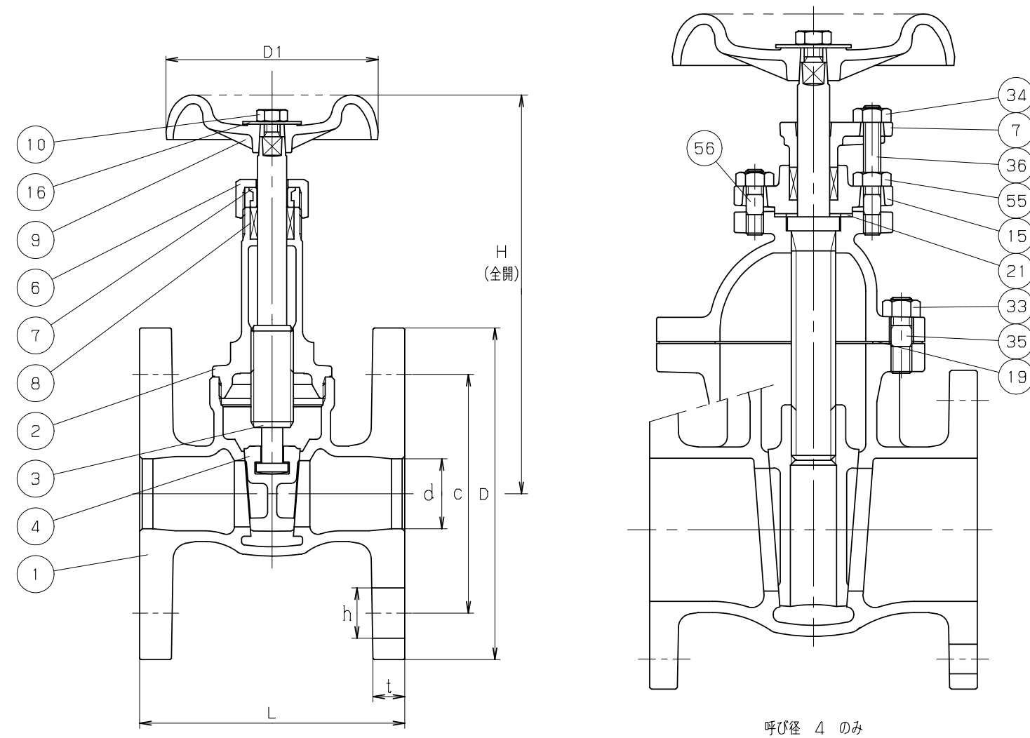
寸法表
