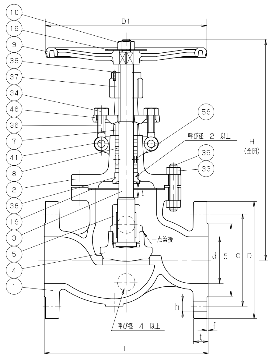
寸法表
