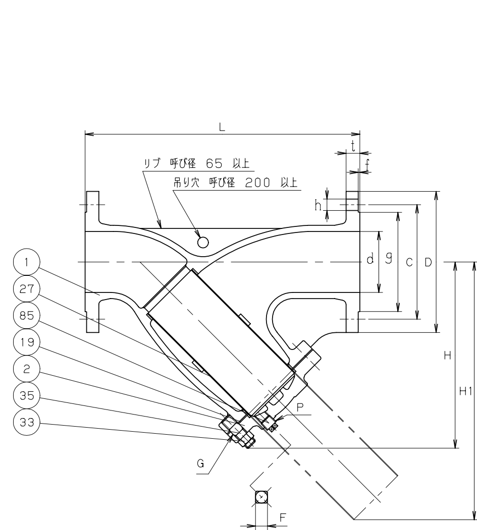
寸法表
