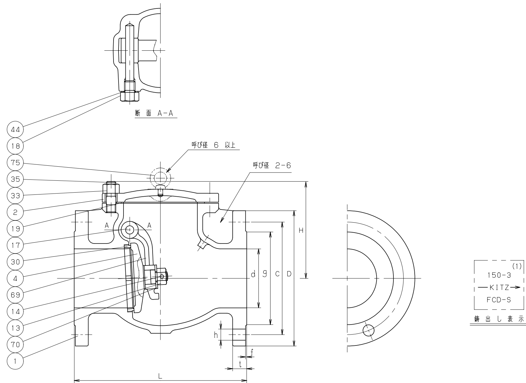
寸法表
