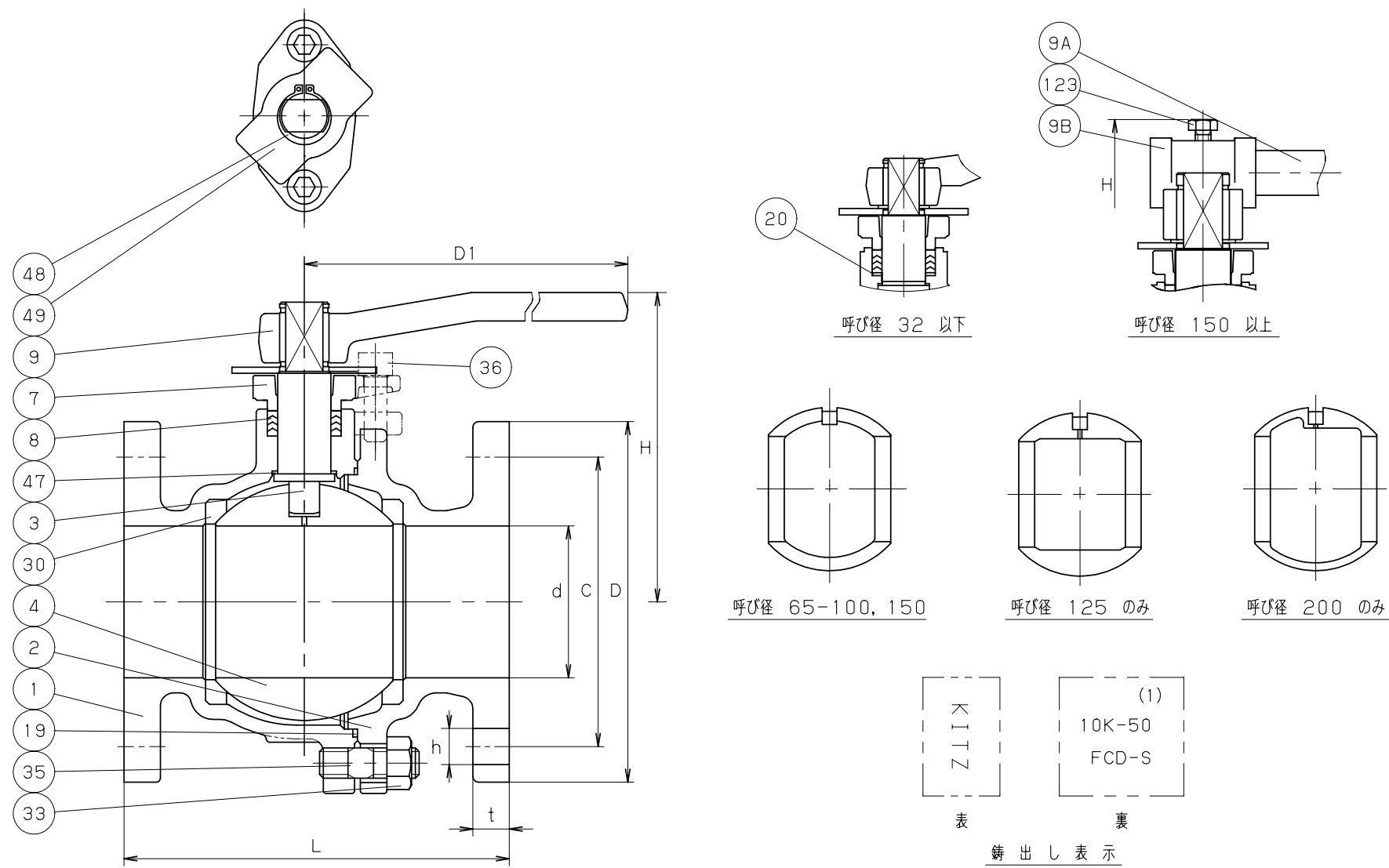
寸法表
