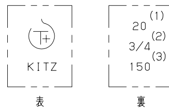
鋳出し表示
