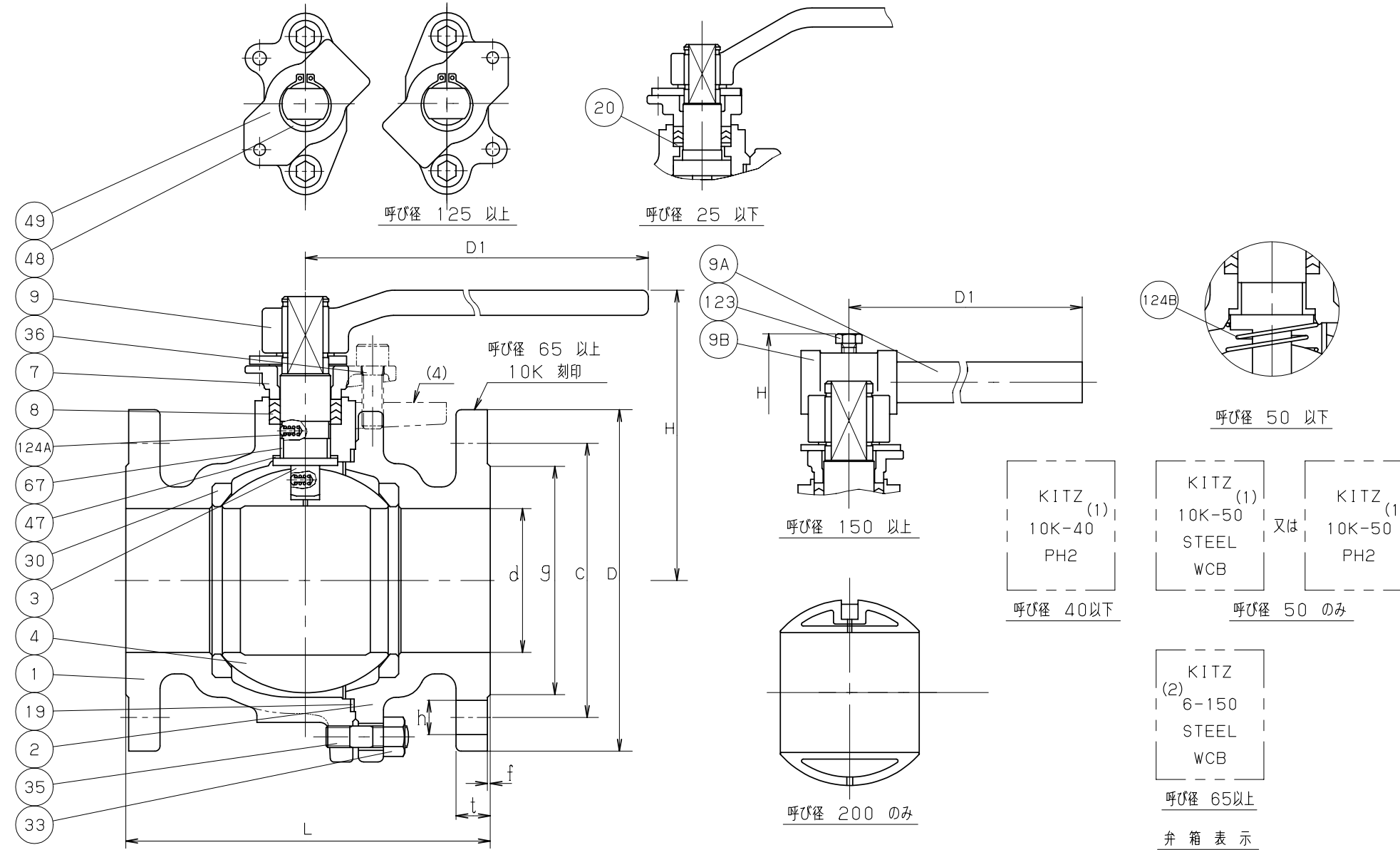
寸法表
