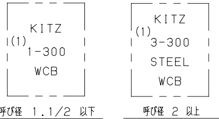
弁箱表示
