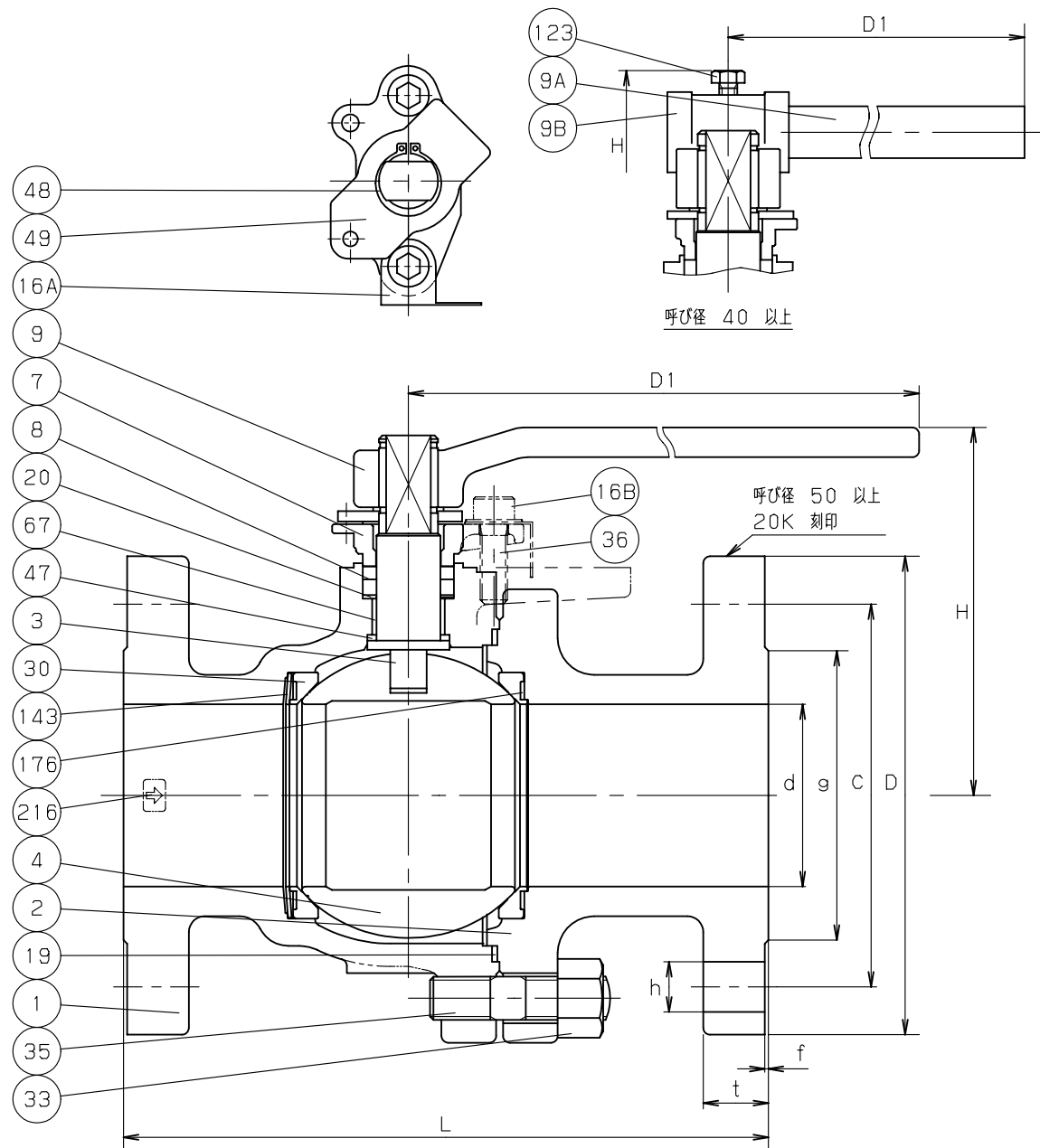
寸法表
