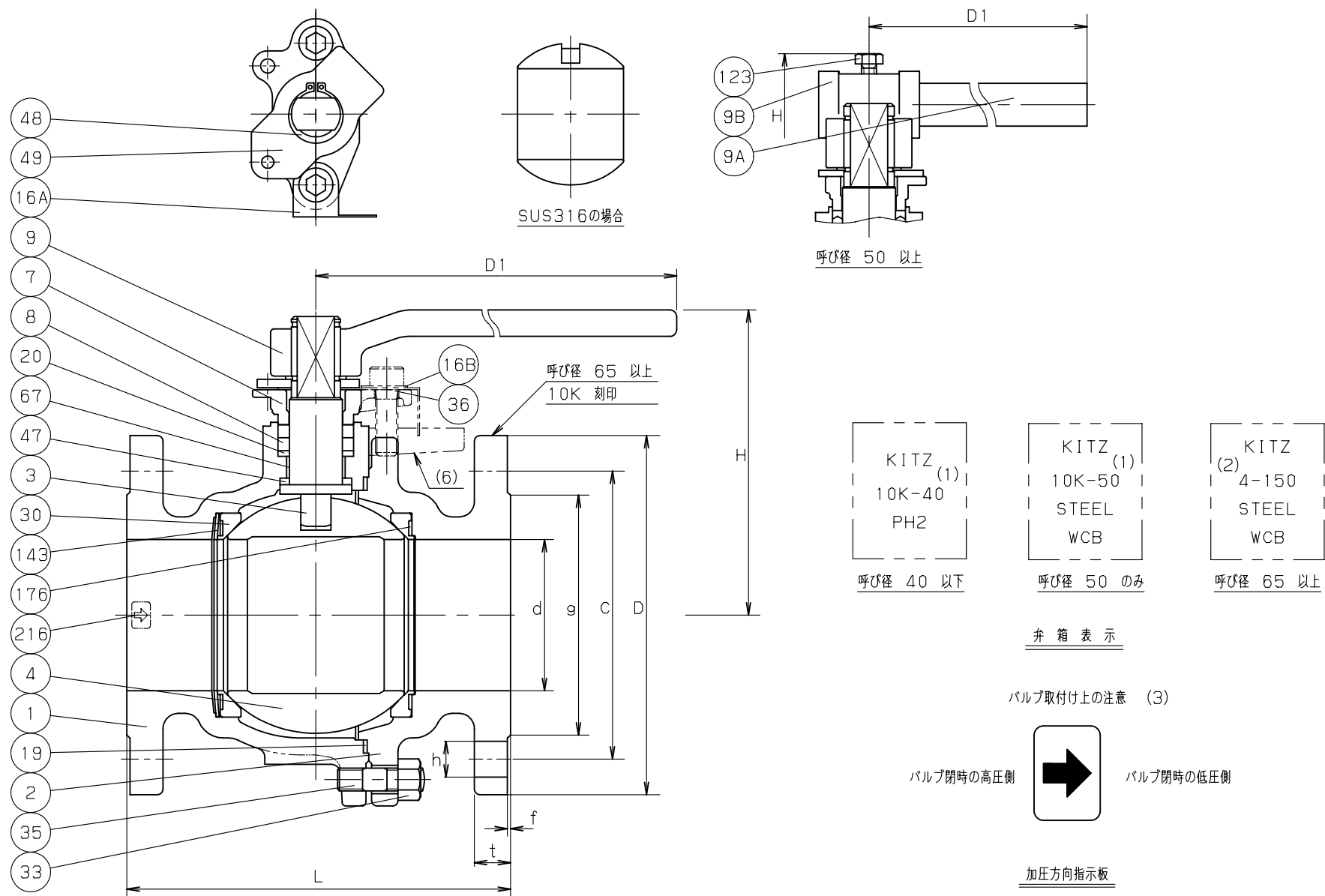
寸法表
