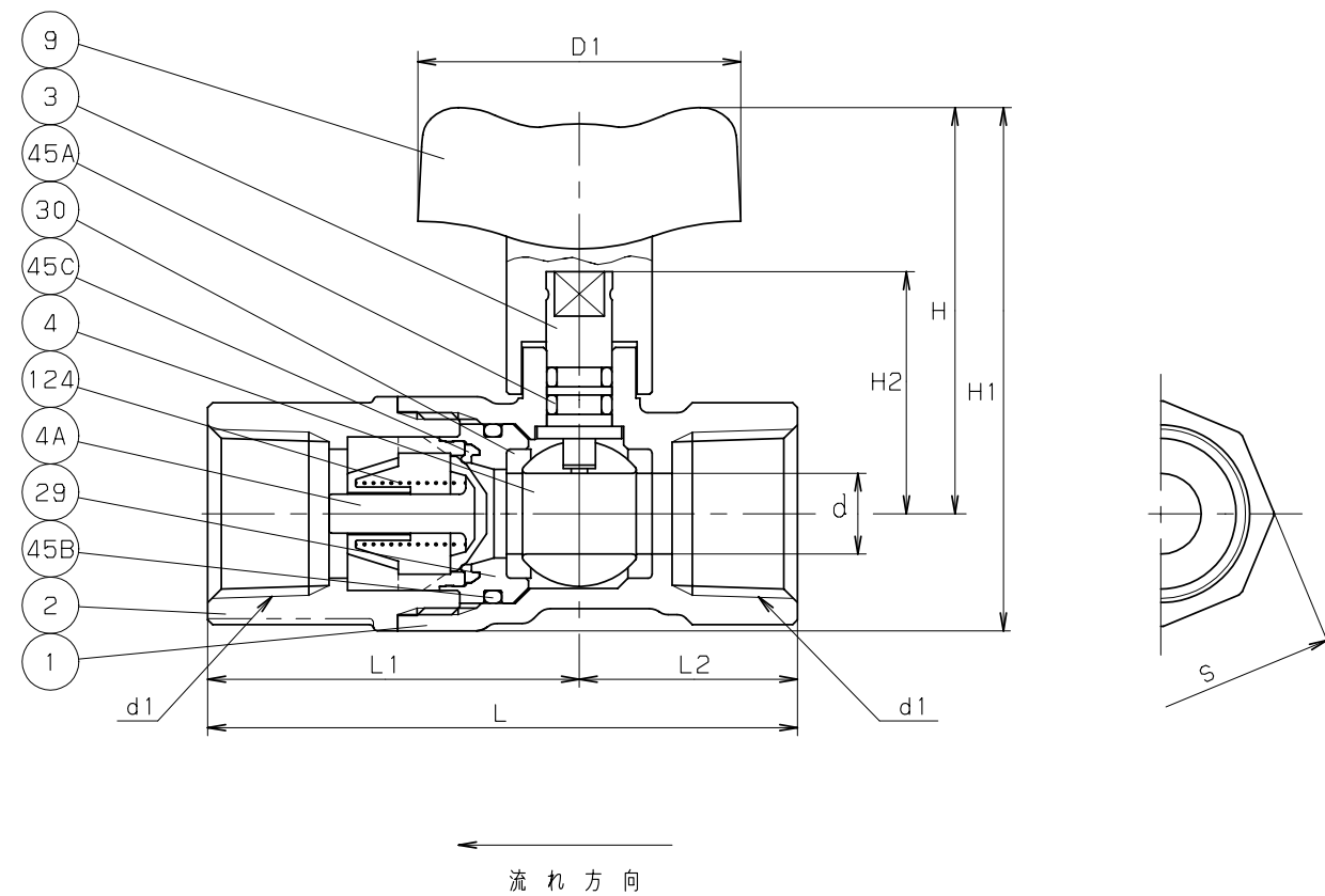
寸法表
