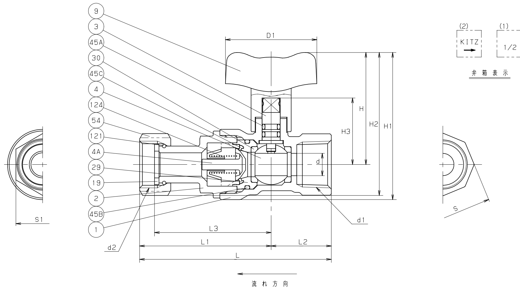
寸法表
