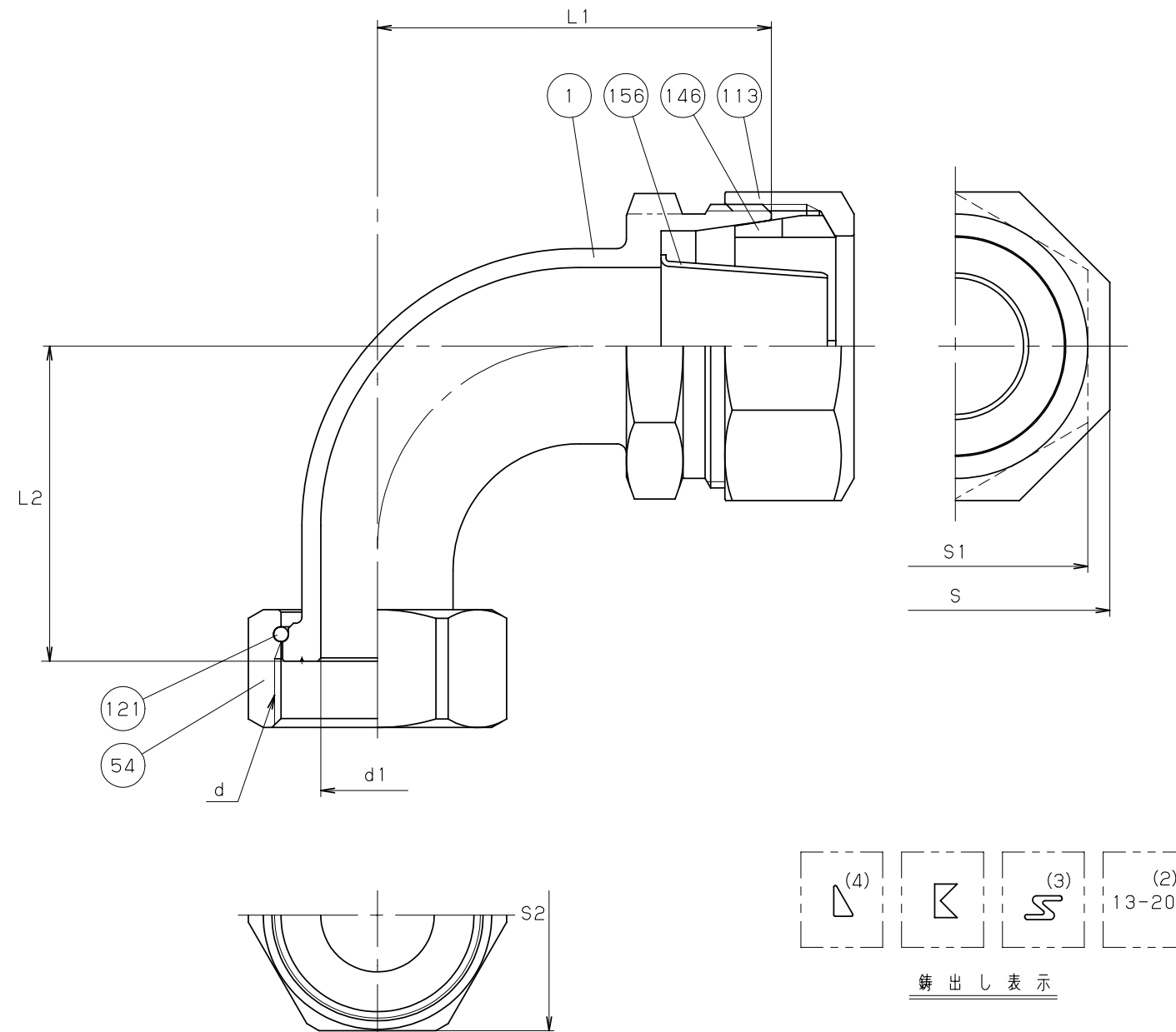
寸法表
