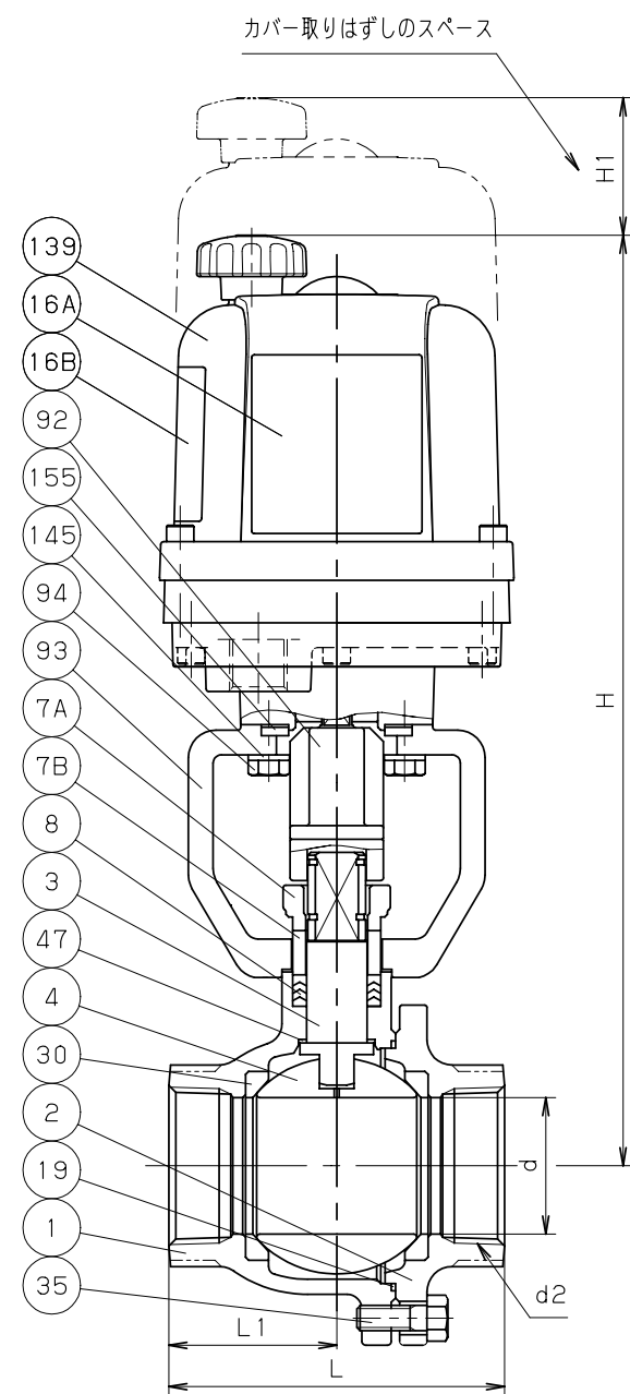
寸法表
