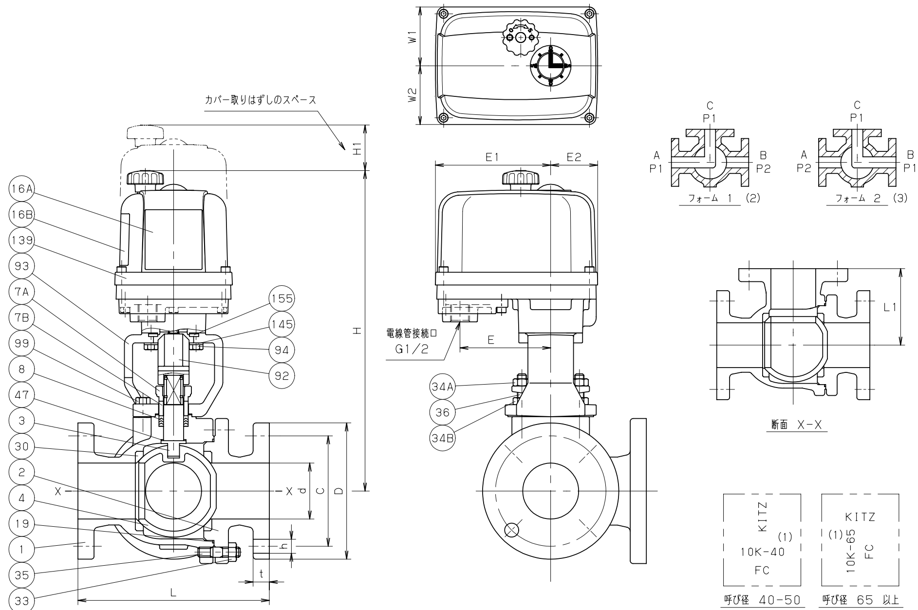
寸法表
