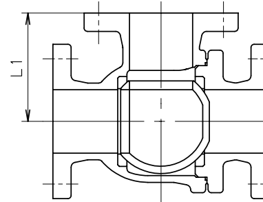
断面 X-X
