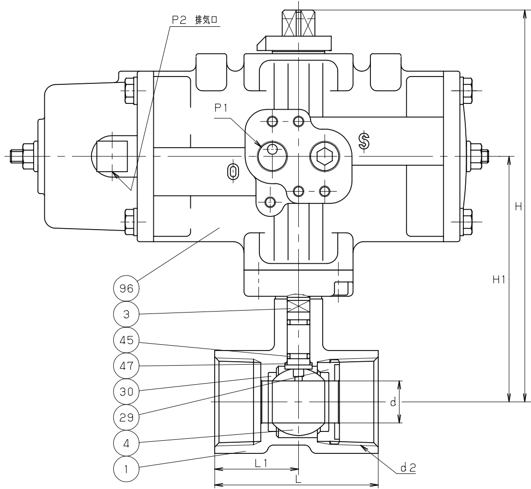
寸法表
