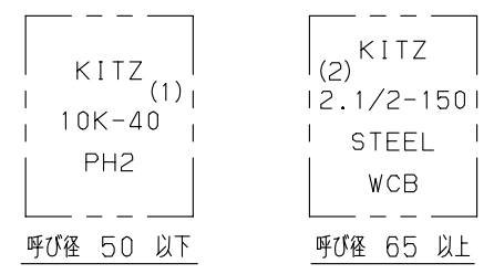
弁箱表示
