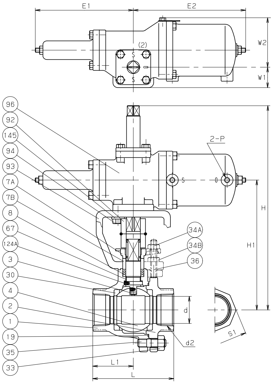
寸法表
