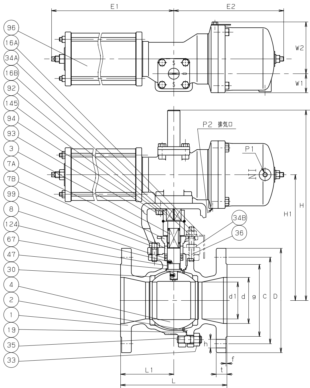
寸法表
