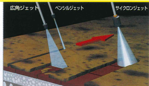
サイクロンジェットノズル/ペンシルジェット(0°)を高速で回転させるので、広角ジェット(25°~40°)の約10倍もの威力があります。こびりついた汚れの広範囲洗浄に最適です。
