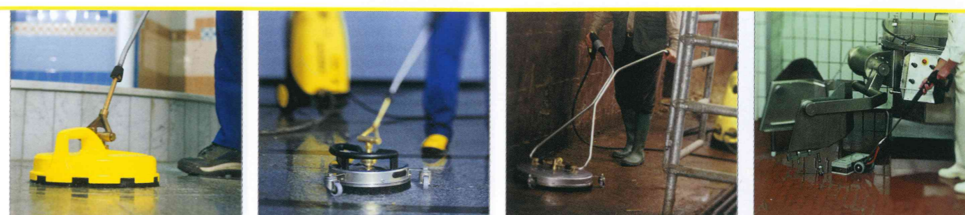
FR 30 P スプレーランスに取付けて水ハネなしで強力に床面の洗浄ができます。 FR 30 Me FR 50 Me フロアクリーニングランス
